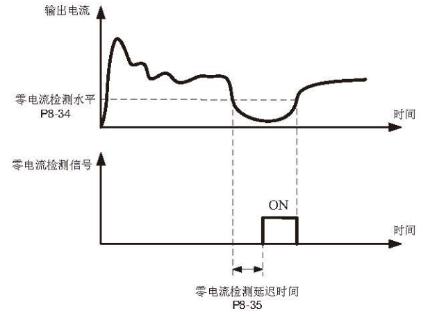
图 6-21 零电流检测示意图
