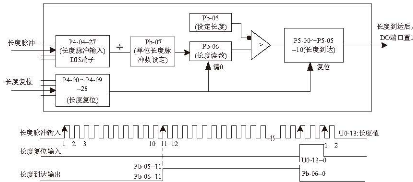
图 4-26 定长控制模式功能码设置
