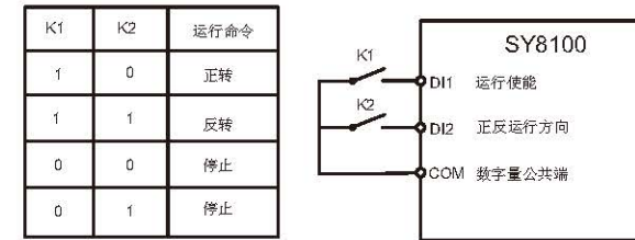
图 6-7 两线式模式 2
