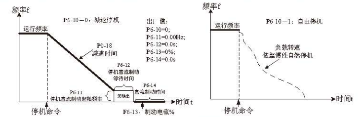
图 4-11 停机模式
