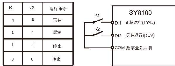
图 6-6 两线式模式 1
