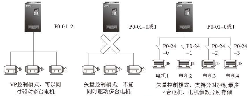
图 4-29 多组电机的切换
