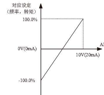
图 6-10 模拟给定与设定量的对应关系
