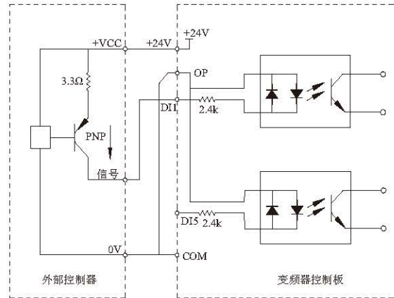
图 3-20 源型接线方式
