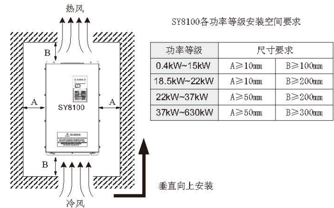
图 3-1 SY8100 变频器各功率等级安装空间要求
