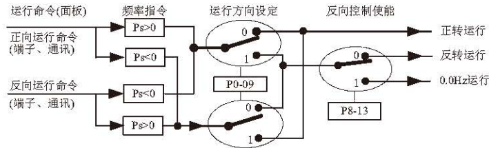
图 4-25 电机运转方向设置
