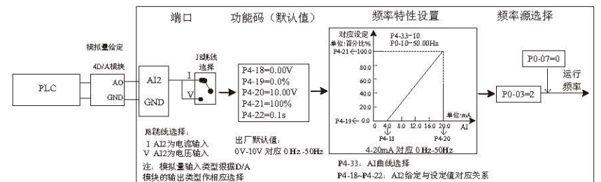
图 4-20 AI2 电流型输入给定频率功能码设置
