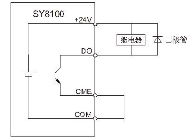
图 3-21 数字输出端子接线示意图
