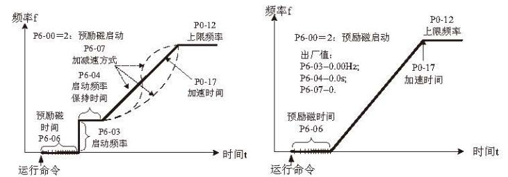
图 4-10 预励磁启动方式
