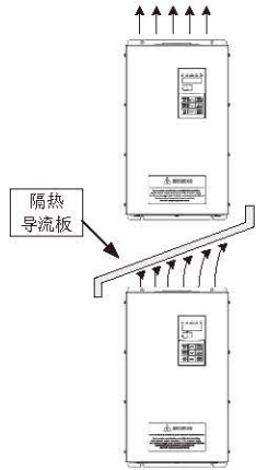
图 3-2 隔热导流板安装示意图上下安装图
