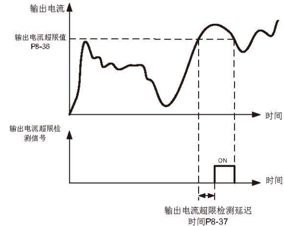
图 6-22 输出电流超限检测示意图
