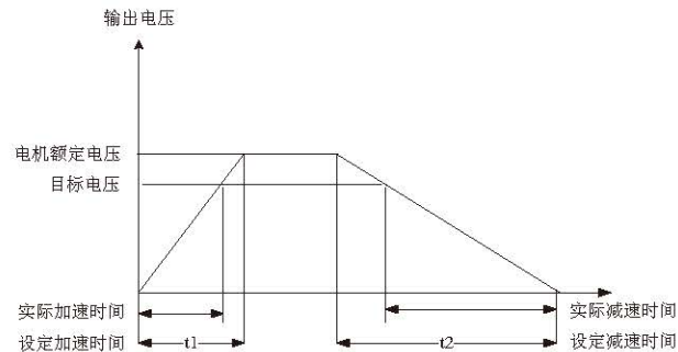
图 6-5 V/F 分离示意图
