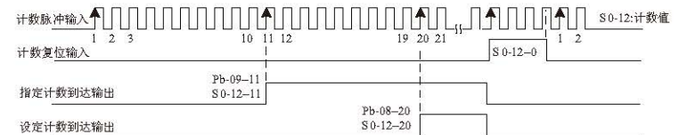
图 6-30 设定计数值给定和指定计数值给定示意图
