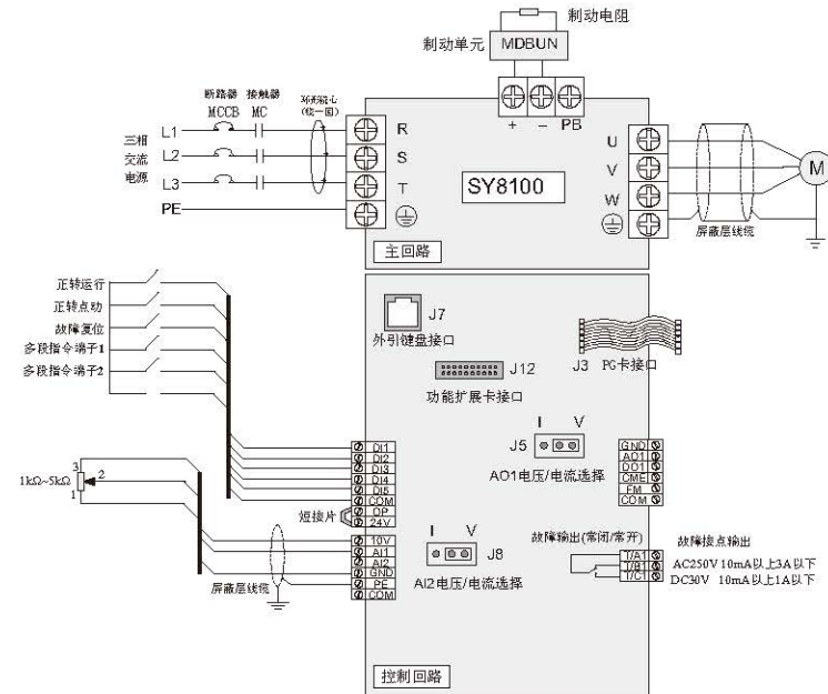
图 3-22 SY8100 电气接线示例
