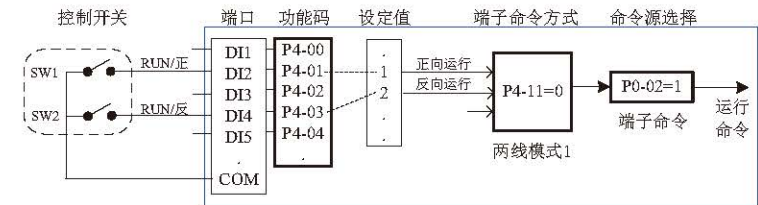
图 4-5 端子启停控制方式举例
