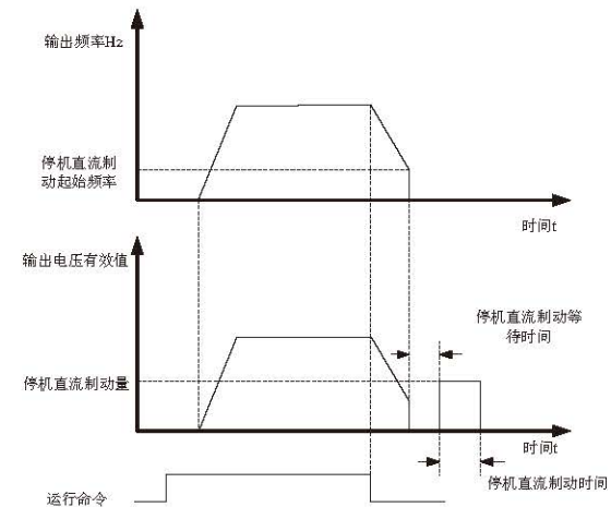
图 6-13 停机直流制动示意图
