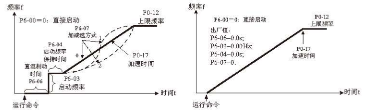
图 4-8 直接启动方式
