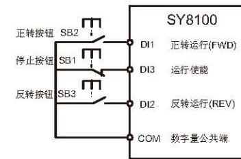
图 6-8 三线式控制模式 1
