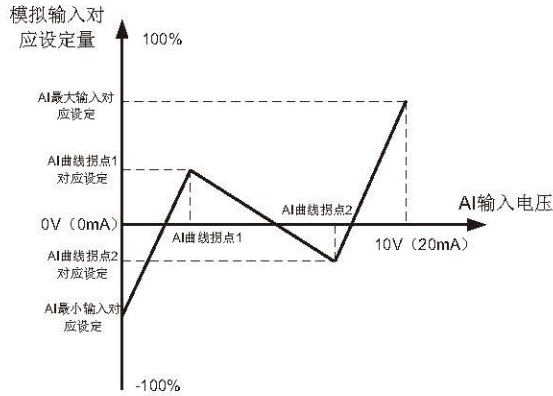
图 6-33 曲线 4 和曲线 5 示意图
