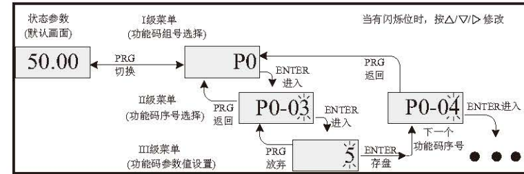
图 4-2 三级菜单操作流程图
