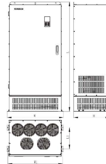
160kw 以上机型的外形尺寸 (380V)
