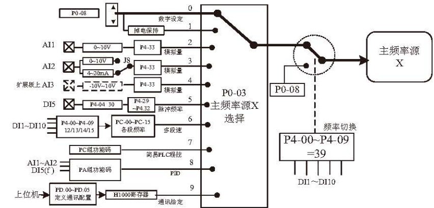
图 4-16 主频率给定来源选择
