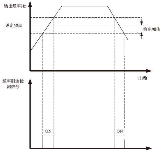
图 6-17 频率到达检出幅值示意图
