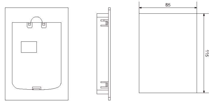
图 7-16 外引键盘的外型尺寸
