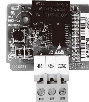
附录 H: 图 1 SY8100TX1 外型图
