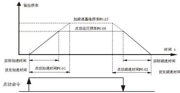
图 4-13 点动运行方式
