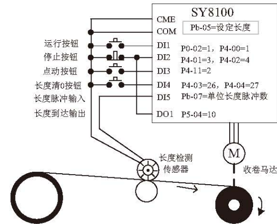
图 4-27 定长控制功能常见应用举例
