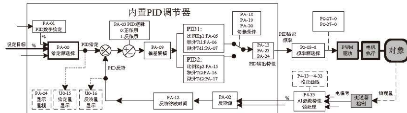
图 4-22 过程控制的频率闭环控制
