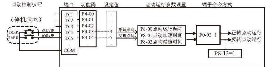
图 4-15 通过 DI 端口点动运行
