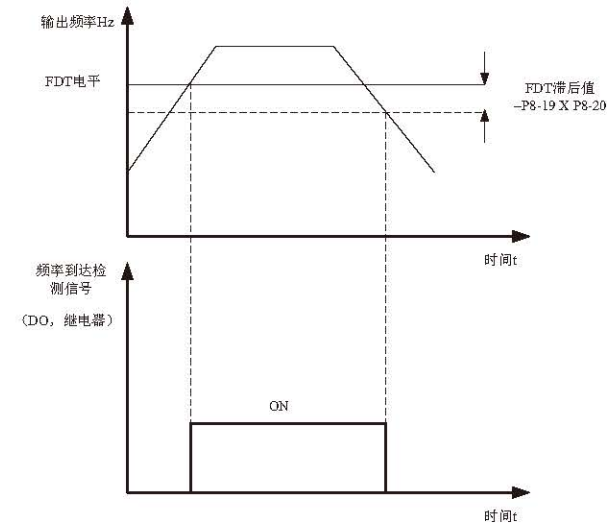
图 6-16 FDT 电平示意图
