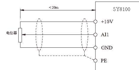
图 3-16 模拟量输入端子接线示意图
