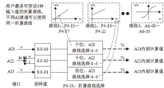
图 4-30 AI 信号对应实际给定
