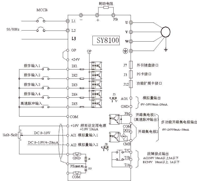
图 3-15 变频器控制回路接线方式
