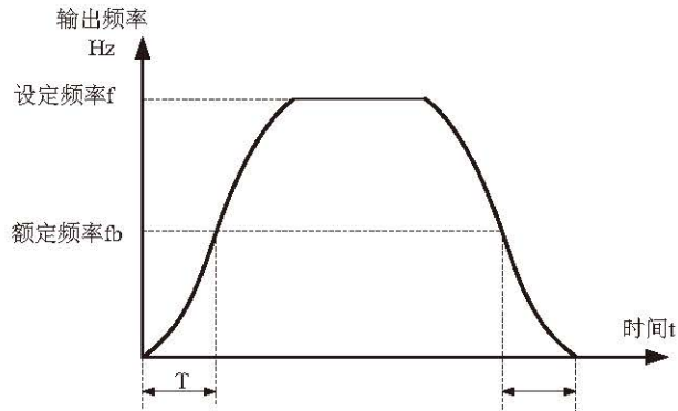
图 6-12 S 曲线加减速 B 示意图
