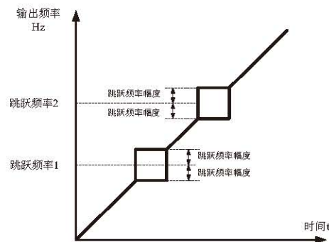
图 6-14 跳跃频率示意图
