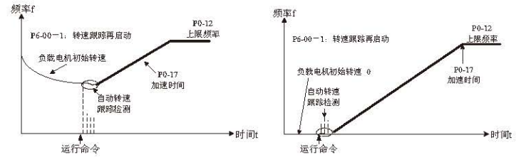
图 4-9 速度跟踪再启动方式
