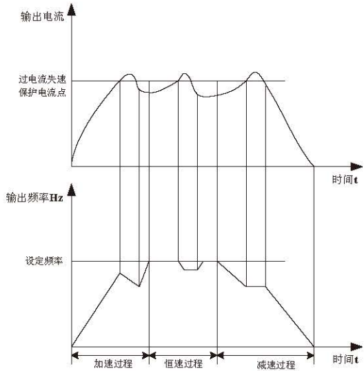
图 6-24 过流失速保护示意图
