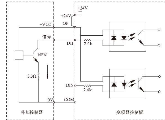
图 3-18 漏型接线方式
