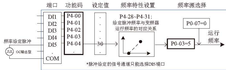
图 4-21 脉冲给定频率功能码设置
