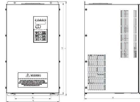
15-132kw 机型外形尺寸 (380V)
