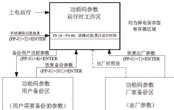
图 4-32 参数备份与恢复设置
