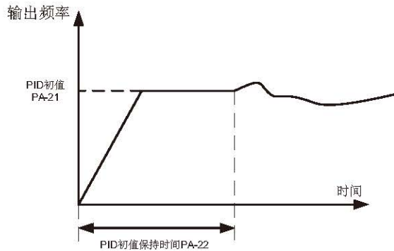
图 6-28 PID 初值功能示意图
