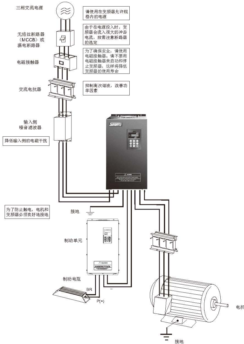
图 2-4 380V 系列系统构成
