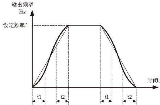
图 6-11 S 曲线加减速 A 示意图
