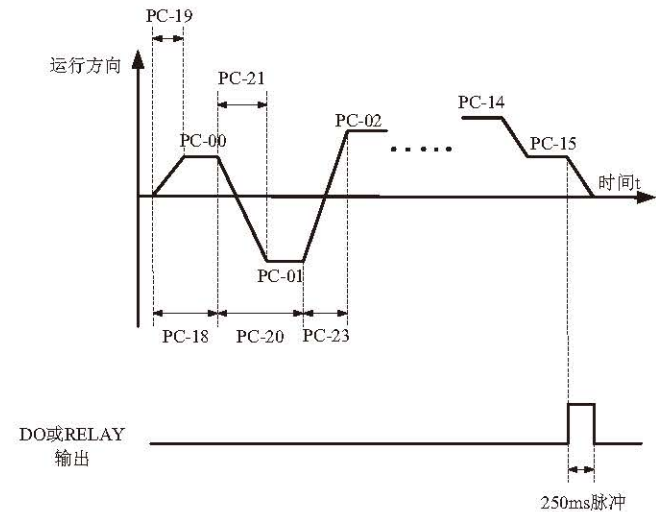
图 6-31 简易 PLC 示意图
